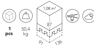
ART. 2889 elemento terminale destro / right end element / angle droit / Abschlusselement rechts / elemento terminal derecho
